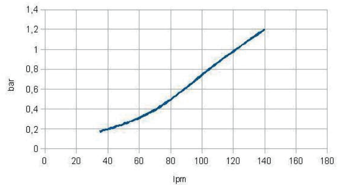
Druckabfall/Pressure Drop
